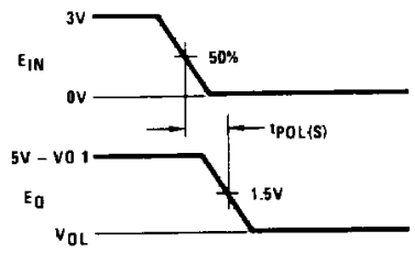
TL/F/5782-16
