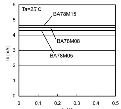
Fig.12 Io - Ib
