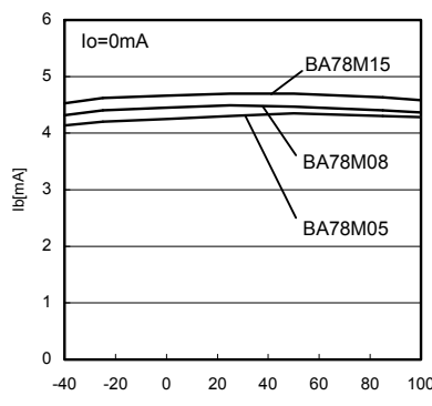
Fig.11 Ta - Ib
