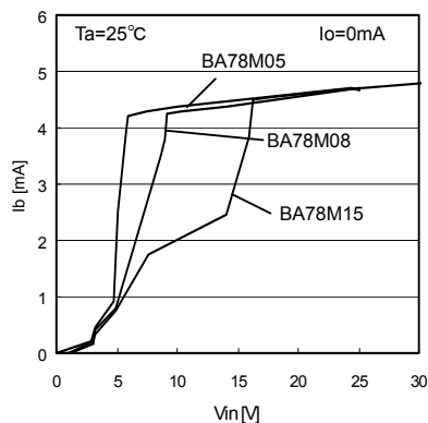
Fig.4 Vin - Ib
