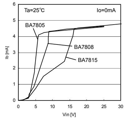
Fig.16 Vin - Ib
