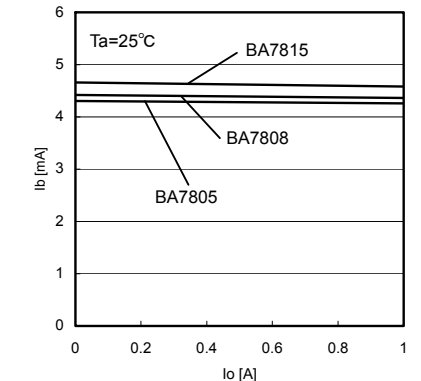
Fig.24 Io - Ib
