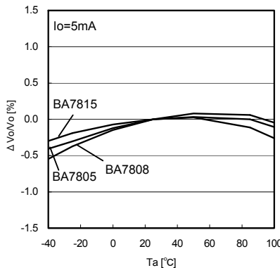
Fig.22 Ta - Vo
