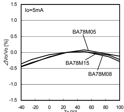
Fig.10 Ta - Vo
