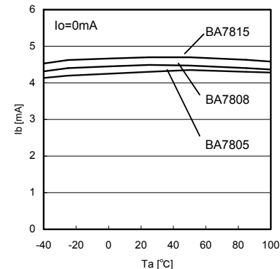
Fig.23 Ta - Ib
