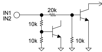
Fig. 20 IN1, IN2 (BA6219BFP-Y, BA6222)
