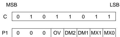
Figure 17. OVLAY parameters
