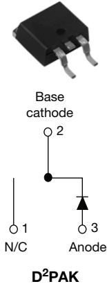
D 2 PAK
