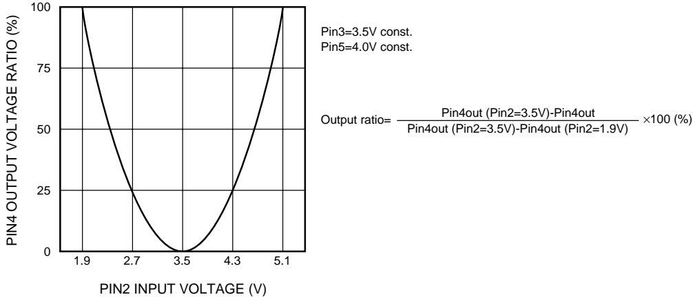
V PARA DC OUTPUT VOLTAGE RATIO
