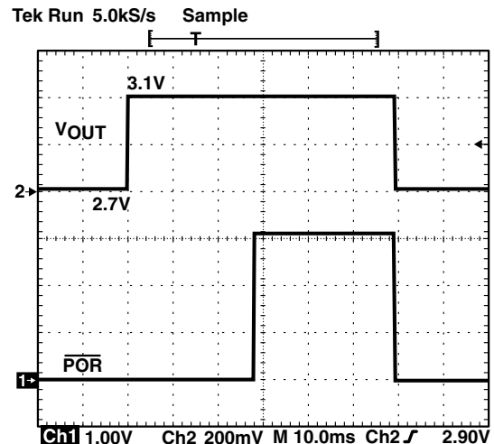
Figure 10. POR Response
