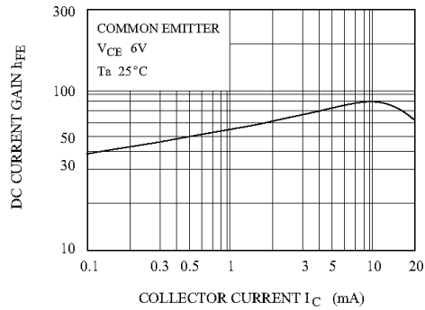
h_{FE} - I_C
