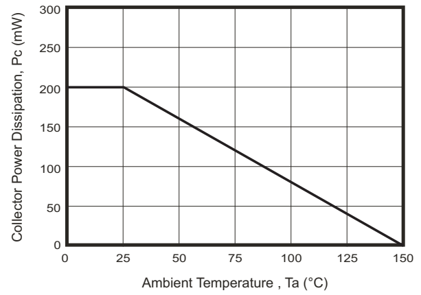
Fig. 8- P_C — T_a
