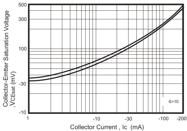
Fig. 3- V_{CEsat} - I_C
