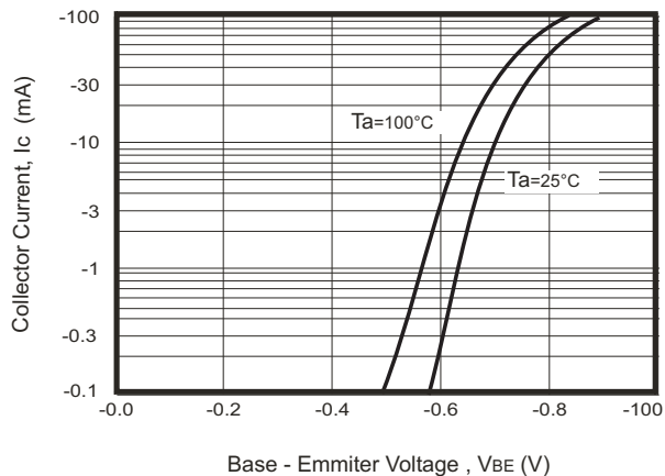
Fig. 5- I_C - V_{BE}
