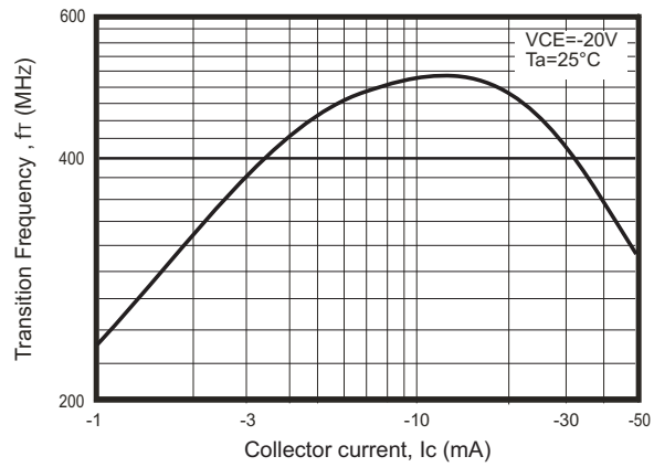
Fig. 7- f_T — I_C
