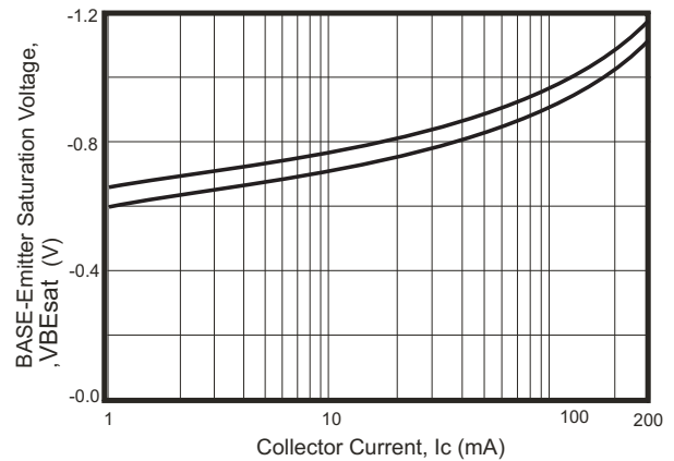
Fig. 4- V_{BEsat} - I_C
