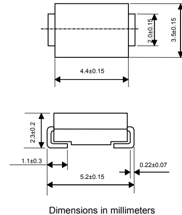
SMB / DO-214AA
