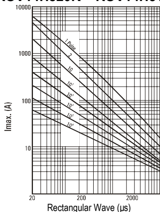
ROV14H820K – ROV14H511K
