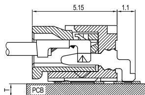
PCB ASS'Y 결합도
