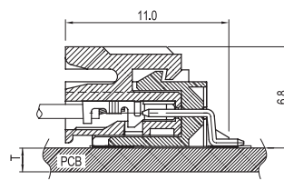
PCB ASS'Y
