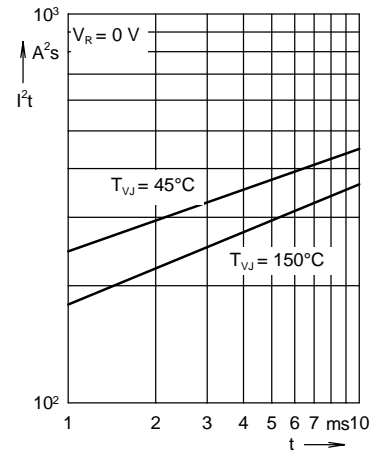
Fig. 3 I^2t versus time per diode
