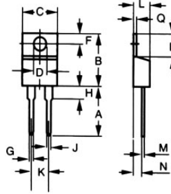
Dimensions TO-220AC
