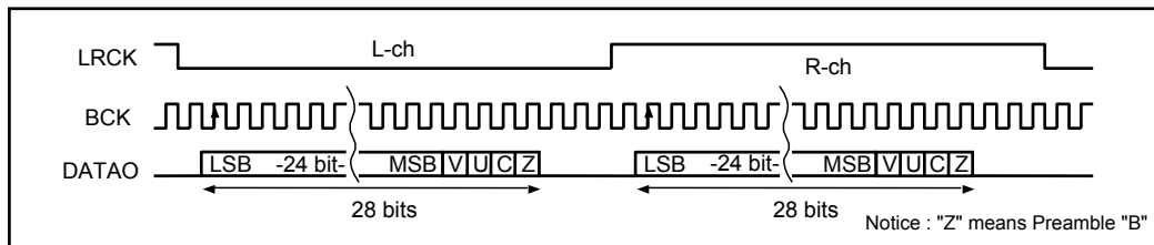
(4) : NRZ data I 2 S output (OFSEL[2 : 0]=110)
