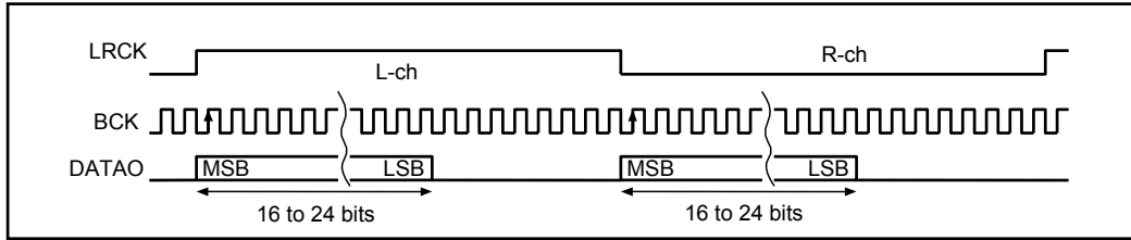
(0) : MSB first left-justified data output (OFSEL[2 : 0]=000)
