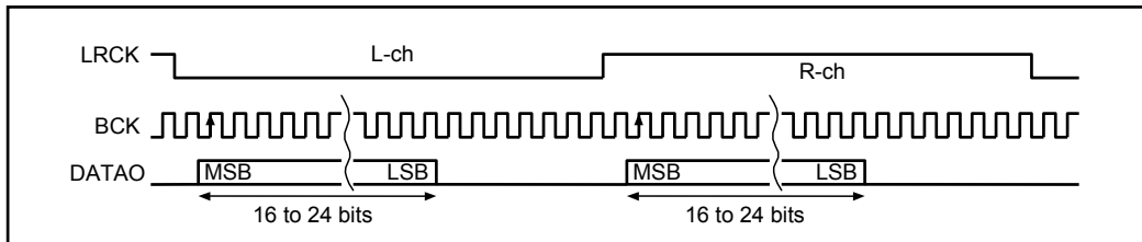
(1) : I 2 S data output (OFSEL[2 : 0]=001)
