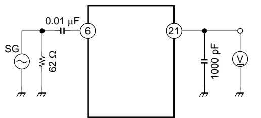
(3) VDATAL
