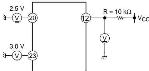
(3) VDATAL
