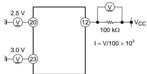
(4) IDATAH
