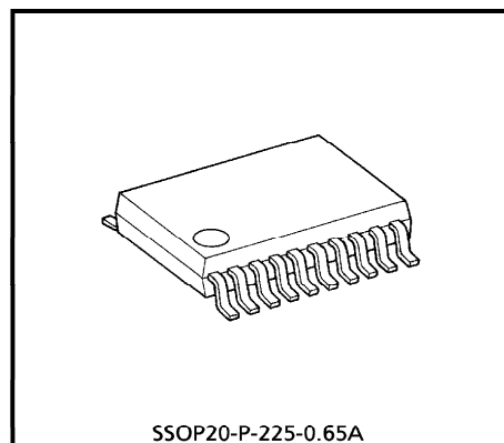
SSOP20-P-225-0.65A
