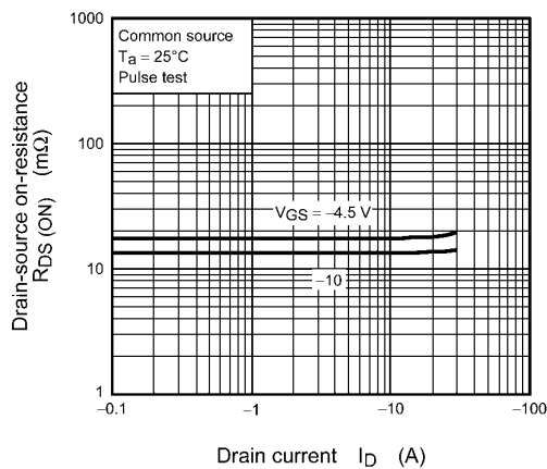
Fig. 8.5 R_{DS(ON)} - I_D
