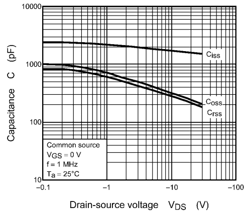
Fig. 8.8 Capacitance - V_{DS}
