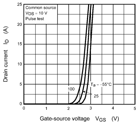
Fig. 8.3 I_D - V_{GS}
