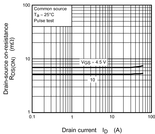
Fig. 8.5 R_{DS(ON)} - I_D
