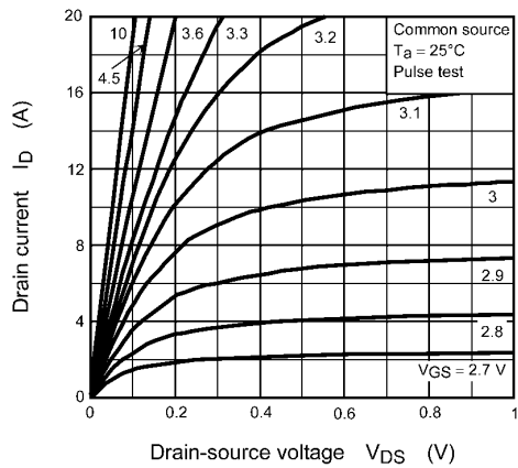
Fig. 8.1 I_D - V_{DS}
