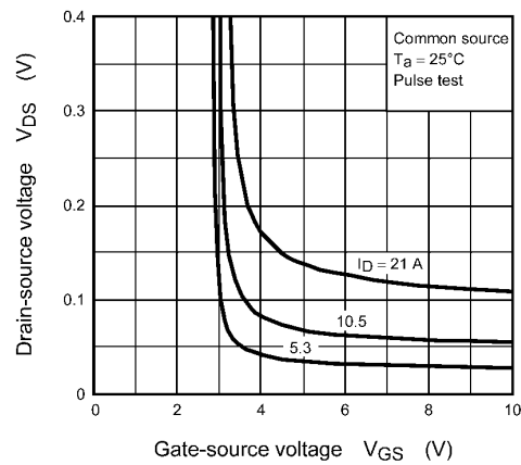
Fig. 8.4 V_{DS} - V_{GS}
