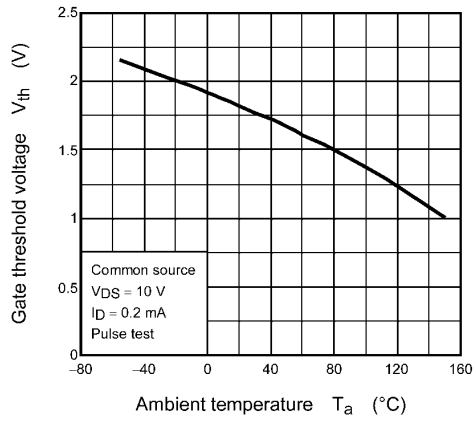
Fig. 8.9 V_{th} - T_a
