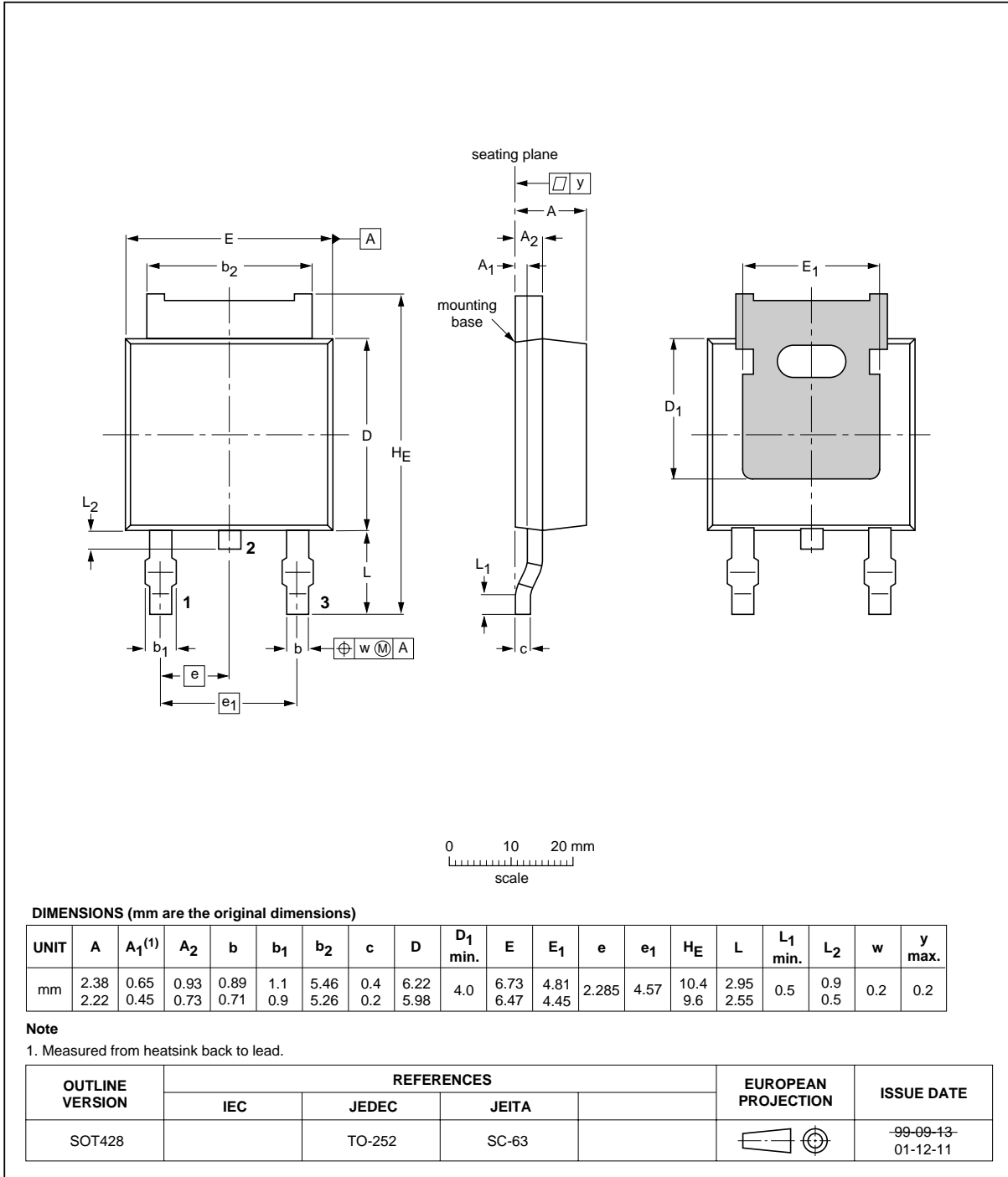
Fig 16. SOT428 (D-PAK).
