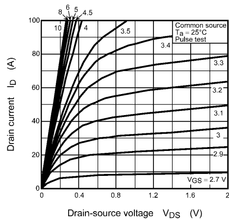
Fig. 8.2 I_D - V_{DS}
