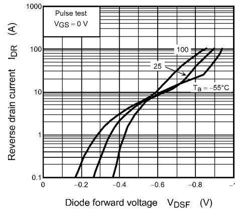
Fig. 8.15 I_{DR} - V_{DSF}
