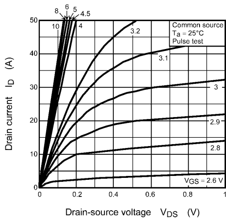
Fig. 8.1 I_D - V_{DS}
