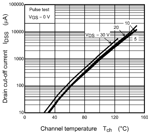
Fig. 8.16 I_{DSS} - T_{ch}
