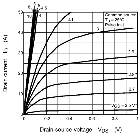
Fig. 8.1 I_D - V_{DS}
