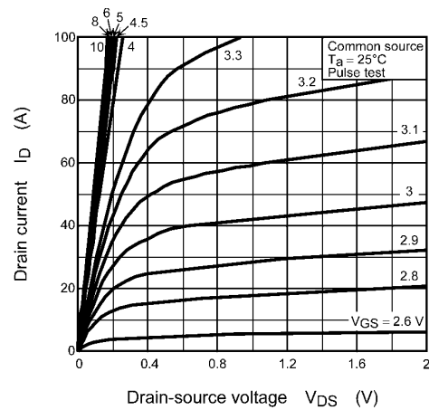
Fig. 8.2 I_D - V_{DS}
