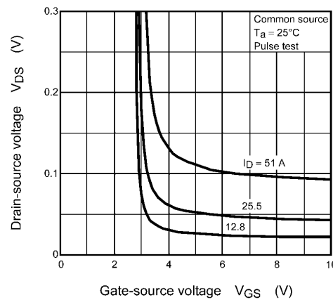
Fig. 8.4 V_{DS} - V_{GS}
