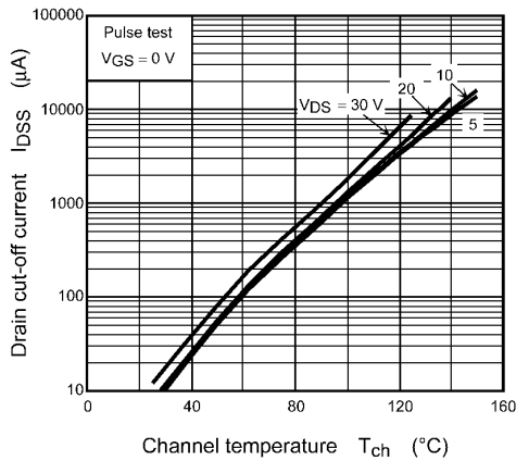
Fig. 8.16 I_{DSS} - T_{ch}
