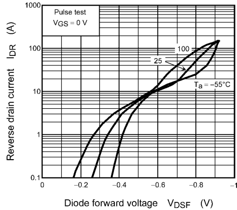
Fig. 8.15 I_{DR} - V_{DSF}
