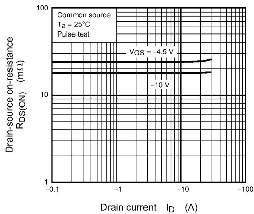
Fig. 8.1.5 R_{DS(ON)} - I_D
