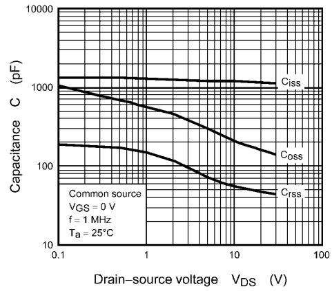
Fig. 8.2.8 Capacitance - V_{DS}
