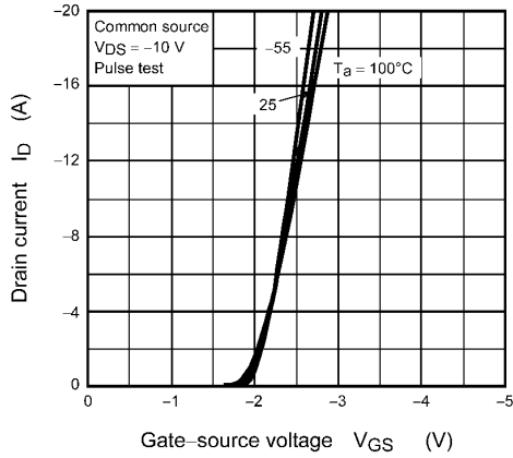
Fig. 8.1.3 I_D - V_{GS}
