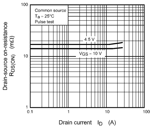
Fig. 8.2.5 R_{DS(ON)} - I_D
