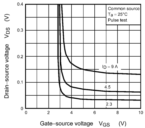
Fig. 8.2.4 V_{DS} - V_{GS}
