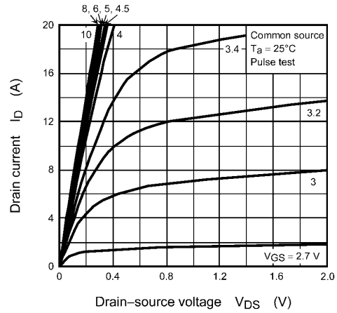
Fig. 8.2.2 I_D - V_{DS}
