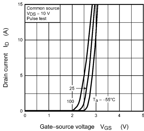
Fig. 8.2.3 I_D - V_{GS}
