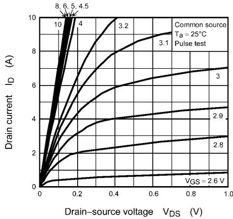
Fig. 8.2.1 I_D - V_{DS}
