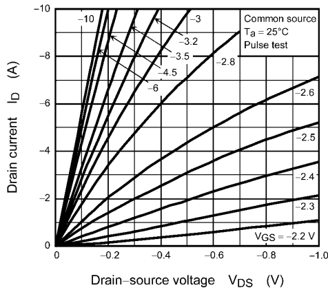
Fig. 8.1.1 I_D - V_{DS}
