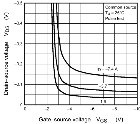
Fig. 8.1.4 V_{DS} - V_{GS}
