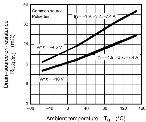
Fig. 8.1.6 R_{DS(ON)} - T_a
