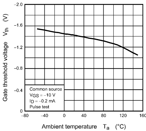
Fig. 8.1.9 V_{th} - T_a
