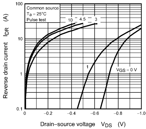
Fig. 8.2.7 I_{DR} - V_{DS}
