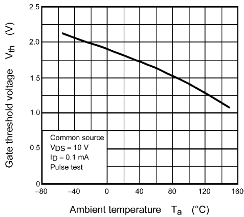
Fig. 8.2.9 V_{th} - T_a
