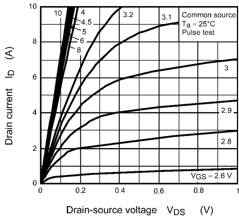
Fig. 8.1 I_D - V_{DS}
