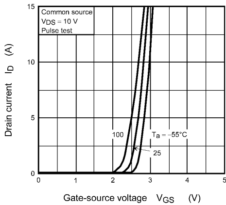
Fig. 8.3 I_D - V_{GS}
