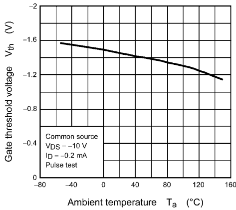
Fig. 8.9 V_{th} - T_a
