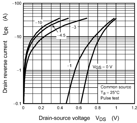
Fig. 8.7 I_{DR} - V_{DS}
