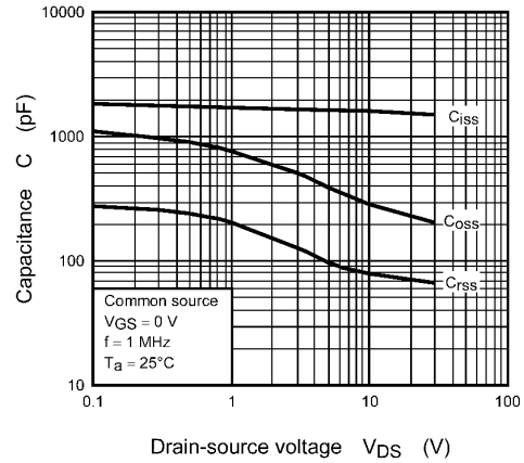
Fig. 8.8 Capacitance - V_{DS}
