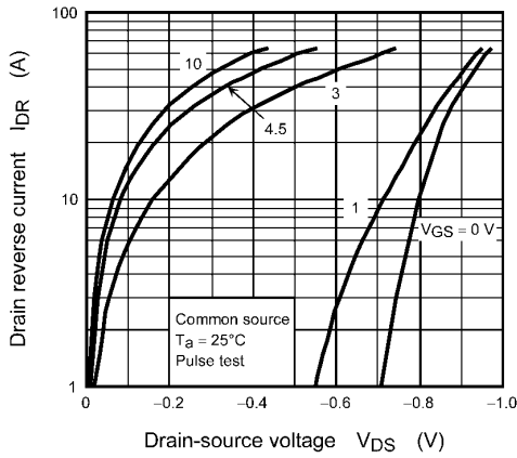
Fig. 8.7 I_{DR} - V_{DS}
