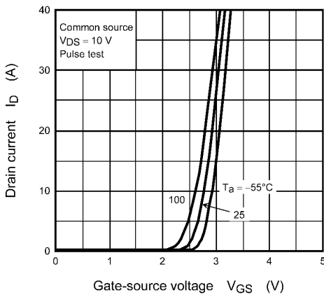
Fig. 8.3 I_D - V_{GS}
