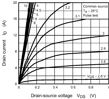
Fig. 8.1 I_D - V_{DS}
