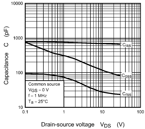
Fig. 8.8 Capacitance - V_{DS}
