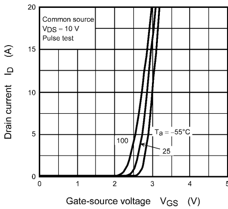
Fig. 8.3 I_D - V_{GS}
