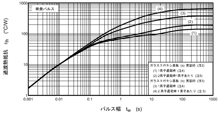
図 8.2.12 r_{th} - t_w (最大値 (保証値))
