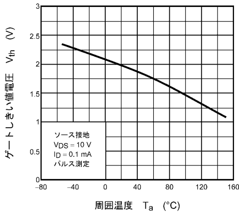
図 8.2.9 V_{th} - T_a
