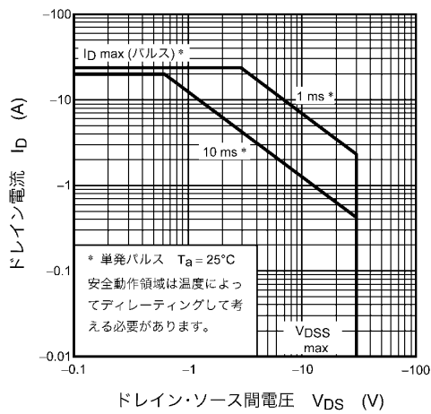
図 8.1.13 安全動作領域 (最大値 (保証値))
