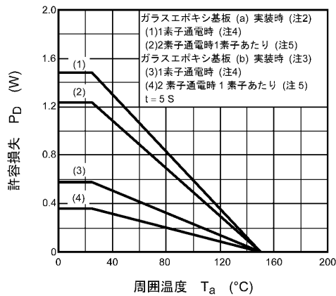
図 8.1.11 P_D - T_a (最大値 (保証値))
