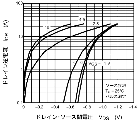
図 8.2.7 I_{DR} - V_{DS}
