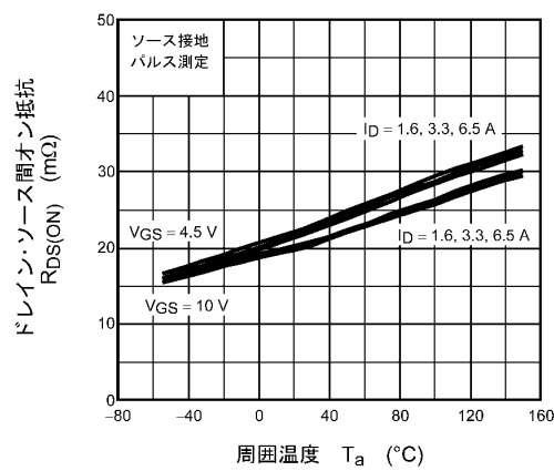
図 8.2.6 R_{DS(ON)} - T_a
