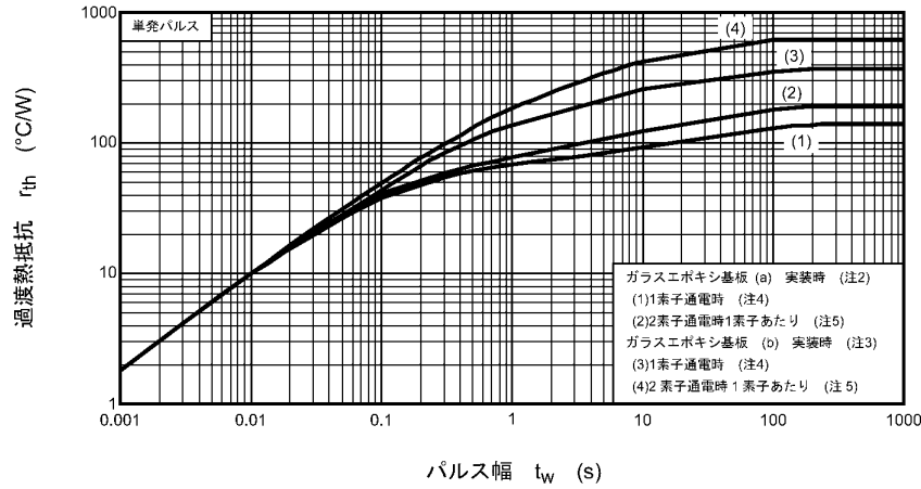
図 8.1.12 r_{th} - t_w (最大値 (保証値))
