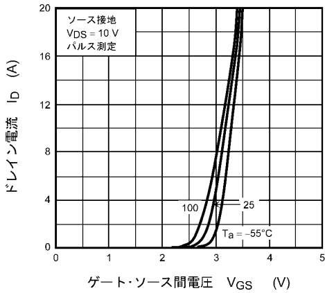
図 8.2.3 I_D - V_{GS}
