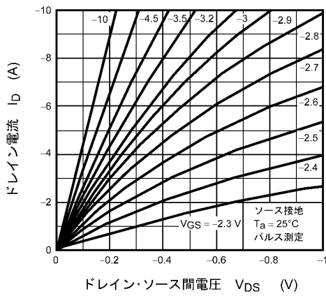
図 8.1.1 I_D - V_{DS}
