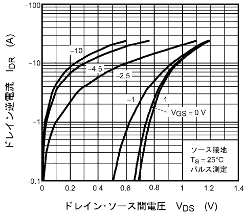
図 8.1.7 I_{DR} - V_{DS}
