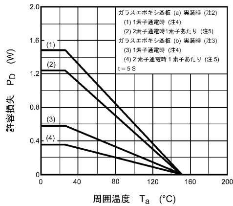
図 8.2.11 P_D - T_a (最大値 (保証値))
