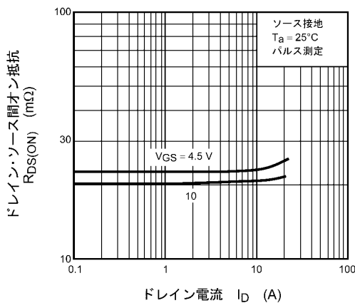
図 8.2.5 R_{DS(ON)} - I_D
