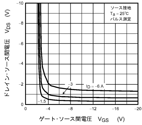
図 8.1.4 V_{DS} - V_{GS}
