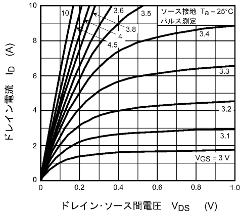
図 8.2.1 I_D - V_{DS}
