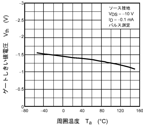
図 8.1.9 V_{th} - T_a
