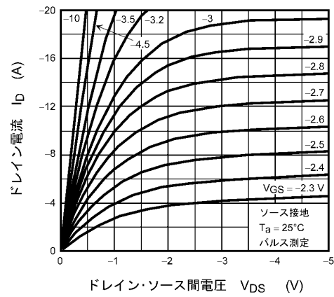
図 8.1.2 I_D - V_{DS}
