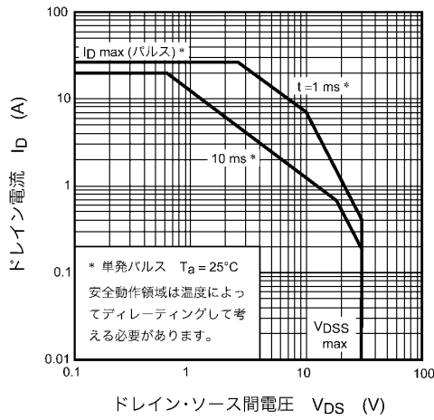
図 8.2.13 安全動作領域 (最大値 (保証値))
