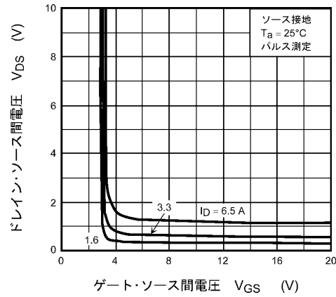
図 8.2.4 V_{DS} - V_{GS}
