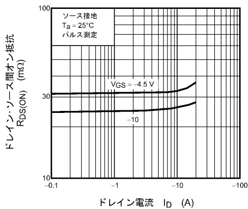
図 8.1.5 R_{DS(ON)} - I_D
