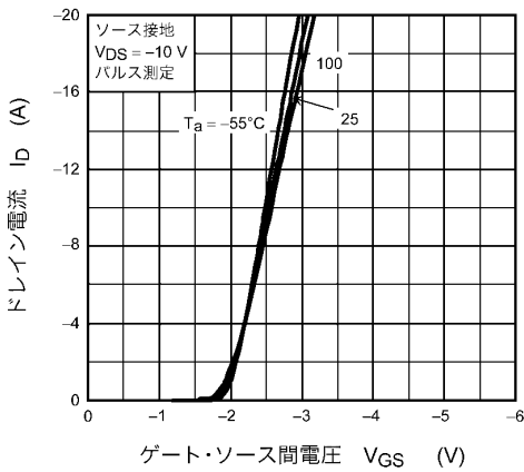
図 8.1.3 I_D - V_{GS}
