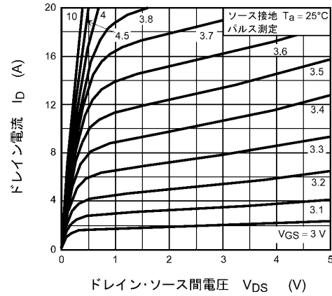
図 8.2.2 I_D - V_{DS}
