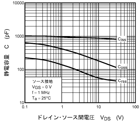
図 8.2.8 静電容量 - V_{DS}
