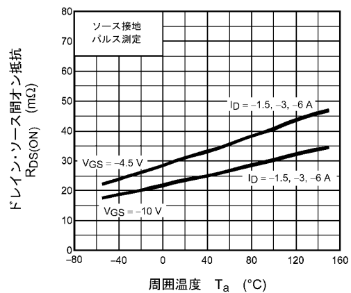
図 8.1.6 R_{DS(ON)} - T_a
