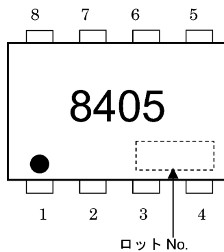
図 7.1 現品表示
