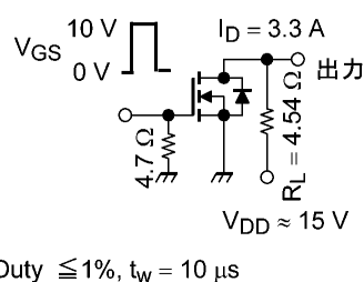
図 6.2.1 スwitchング時間の測定回路例 (P-ch) 図 6.2.2 スwitchング時間の測定回路例 (N-ch)
