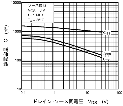
図 8.1.8 静電容量 - V_{DS}
