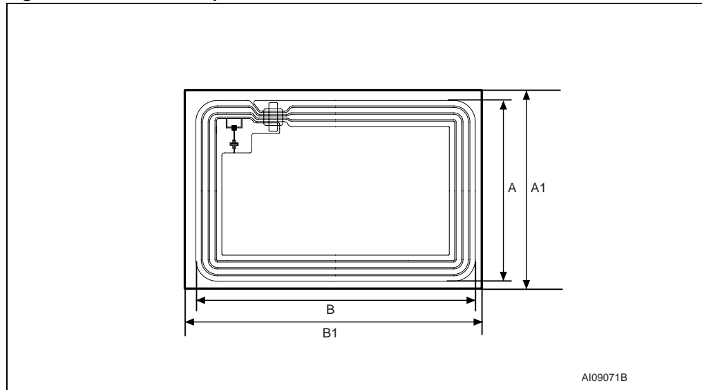
Figure 54. A5 antenna specification
