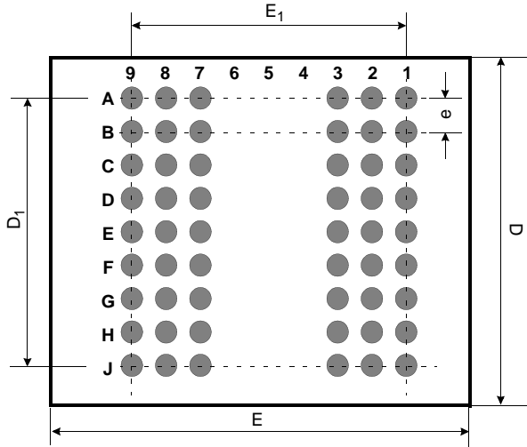
< Bottom View*1 >
