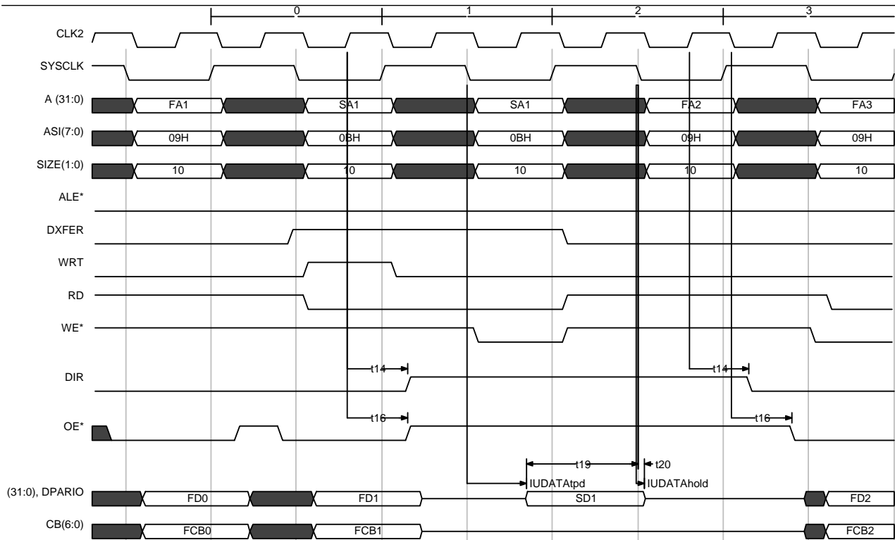
Fig 19) MEC Register Store
