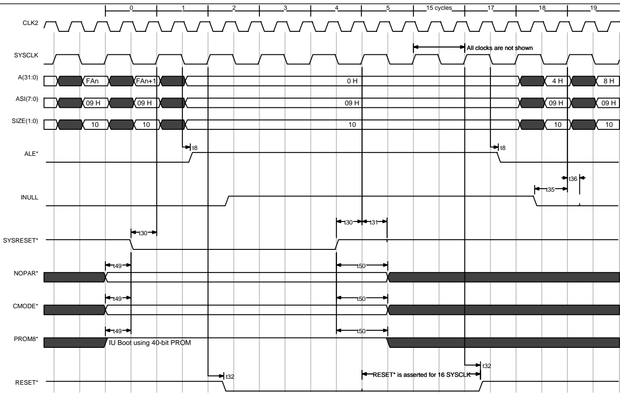
Fig 39) Reset Timing
