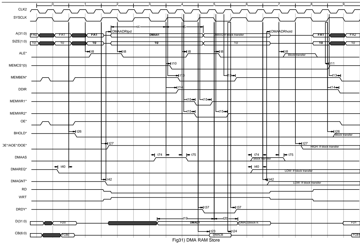
Fig31) DMA RAM Store
