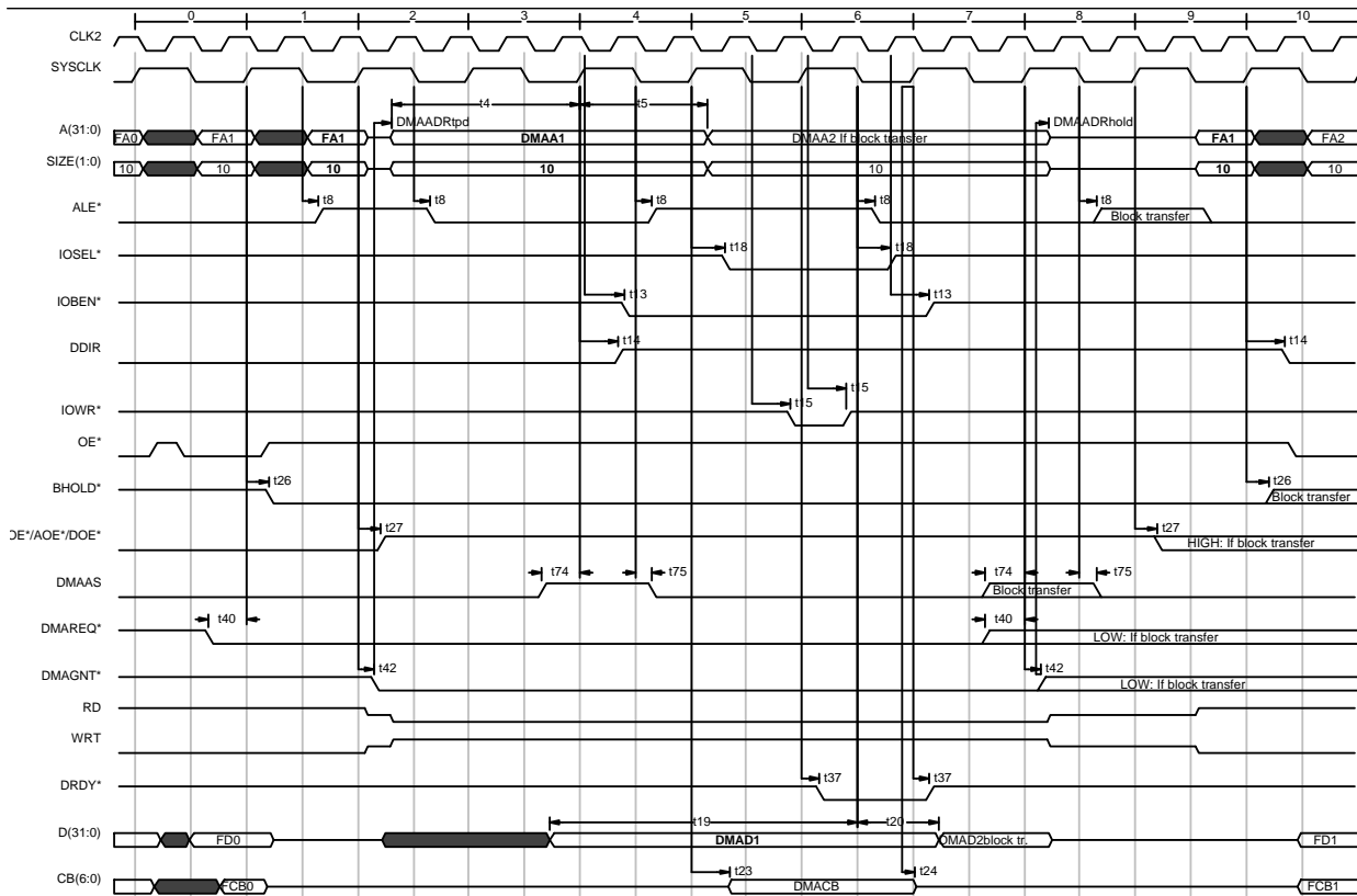
Fig33) DMA IO Store
