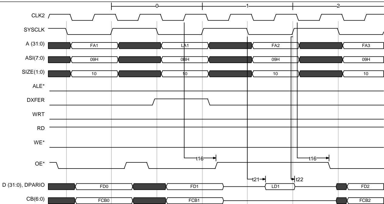
Fig 18) MEC Register Load
