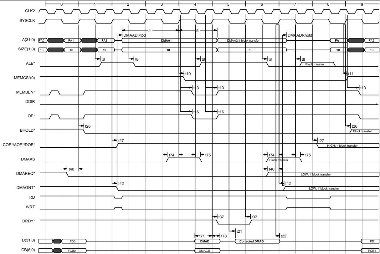
Fig30) DMA RAM Load
