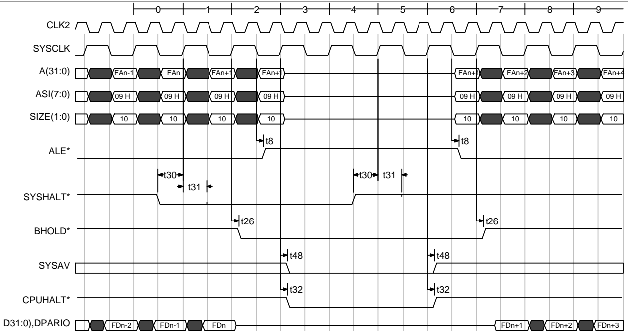
Fig 40) Halt Timing
