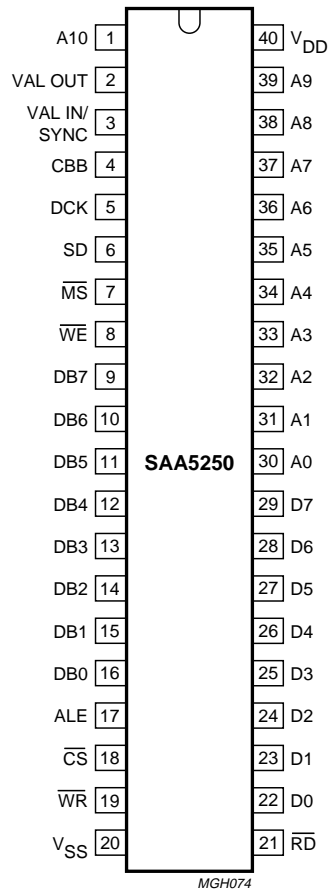
Fig.2 Pinning diagram.
