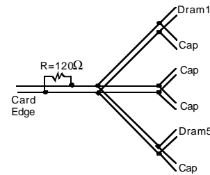
*Clock Net Wiring
