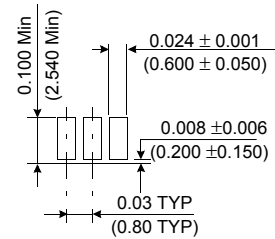
Detail Y
