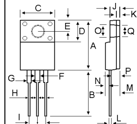
ITO-220AB
