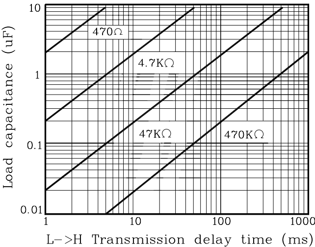
Fig. 9 C_L - t_{PLH}
