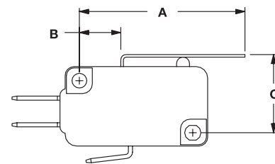
FIG. 3 Lever
