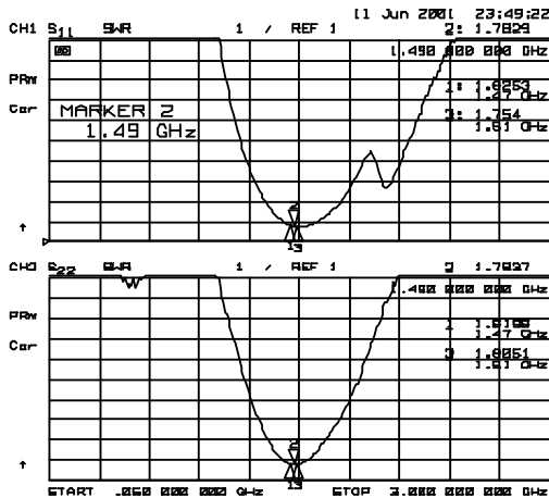
VSWR
