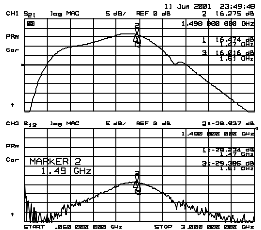
S21, 12
