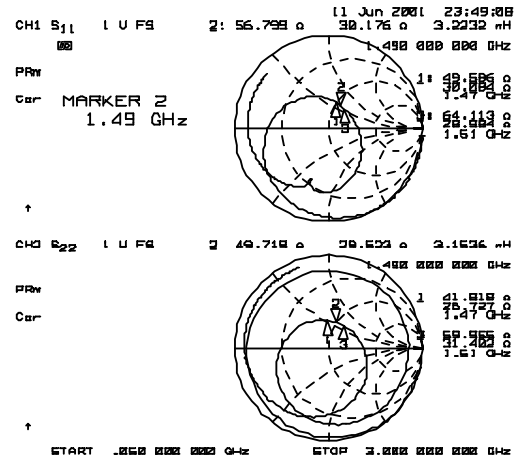
Zin, Zout
