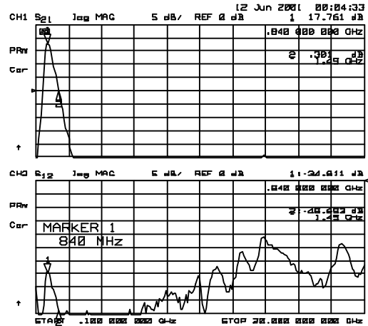
S21, S12
