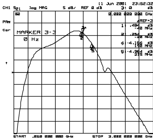
S21
