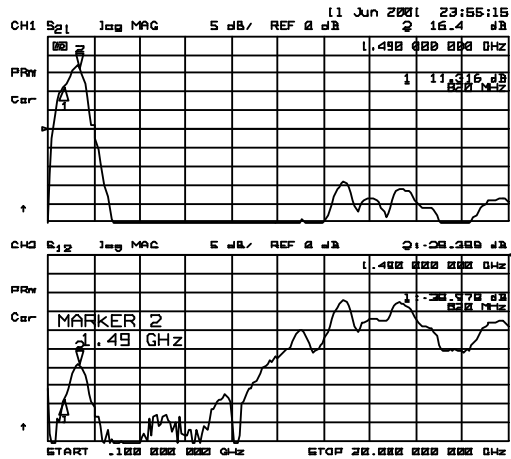
S21, S12
