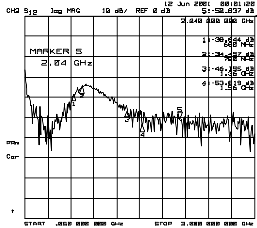
S12
