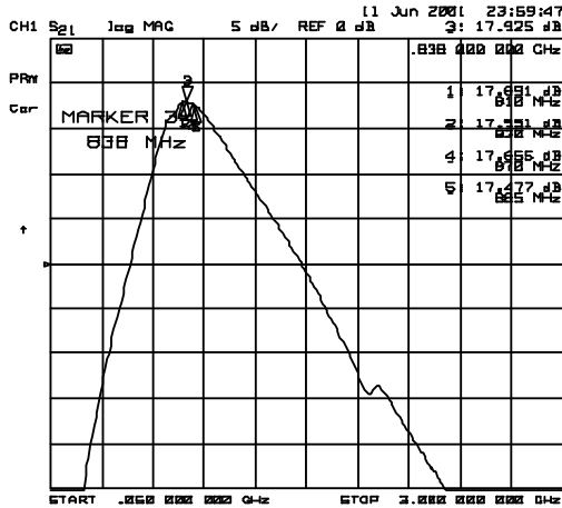
S21
