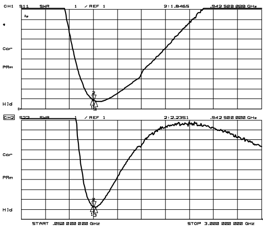
VSWR
