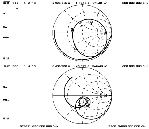
Zin, Zout
