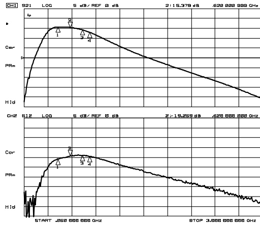
S21, S12
