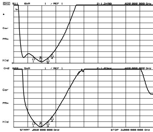
VSWRi, VSWRo
