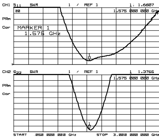
VSWR
