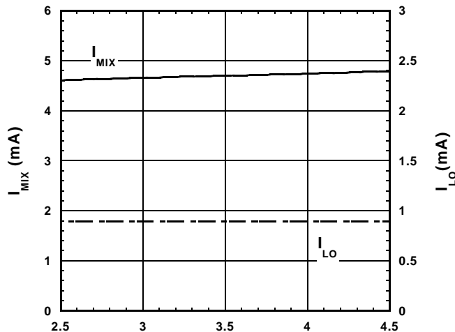
I_{MIX} , I_{LO} vs. V_{MIX} , V_{LO}
