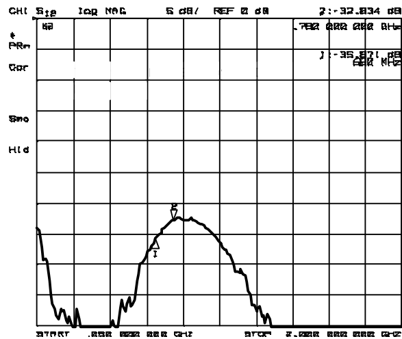
S12
