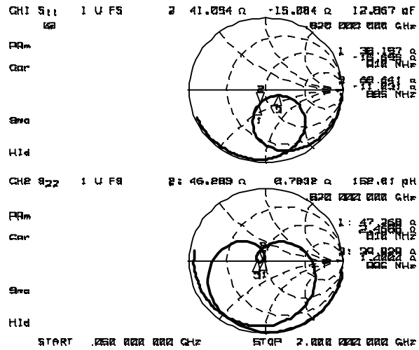
Zin, Zout
