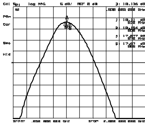
S21
