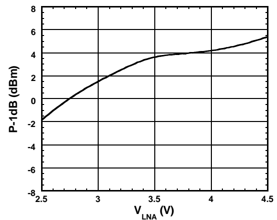
P-1dB vs. V_{LNA} ( f=1900\text{MHz} )
