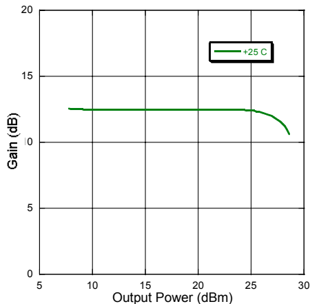
P1dB
