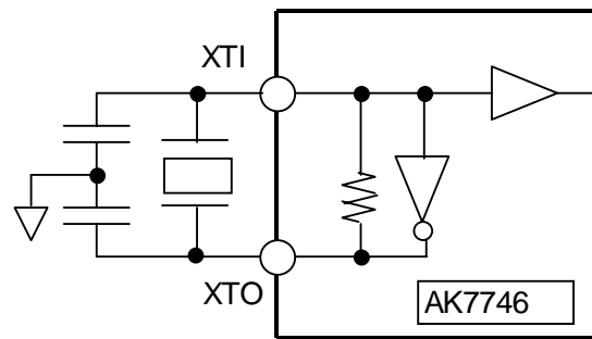
Fig.8-2 Using X'tal : CLK mode 0,1
