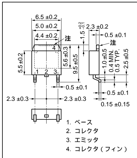
2) TO-252 (MP-3Z)
