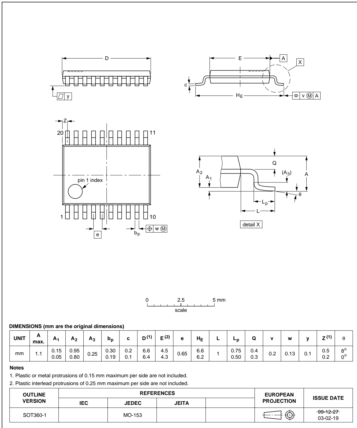
Fig 24. TSSOP20 package outline (SOT360-1)
